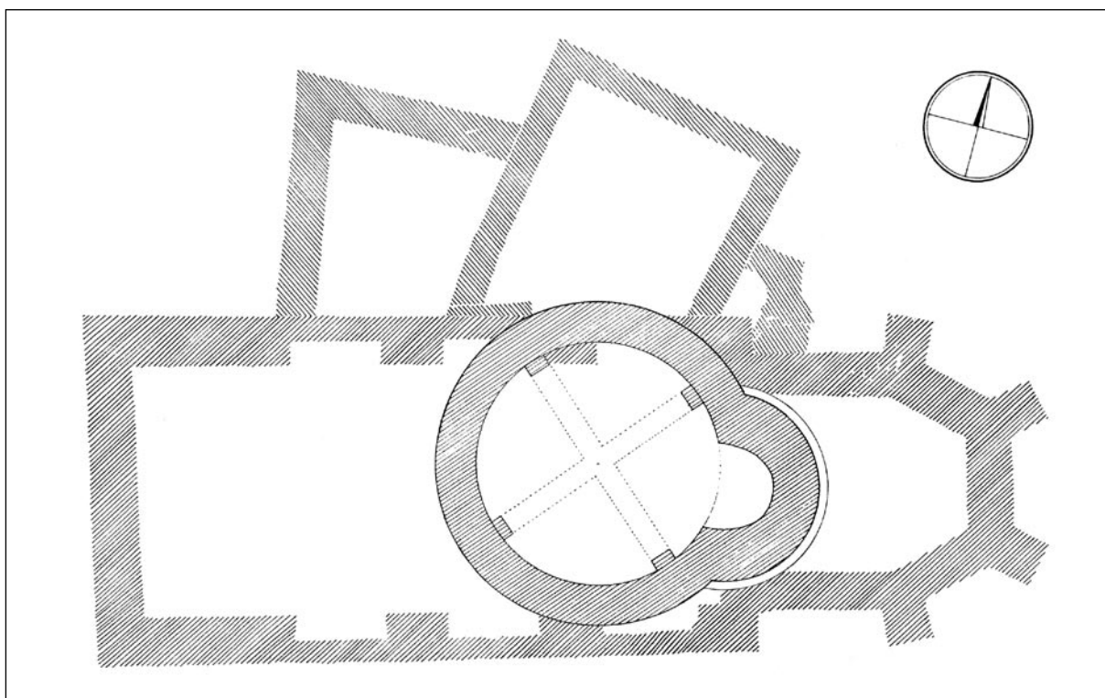
Půdorysná rekonstrukce rotundy z přelomu 11. a 12. století s mladšími přístavbami a s půdorysem gotické stavby.
